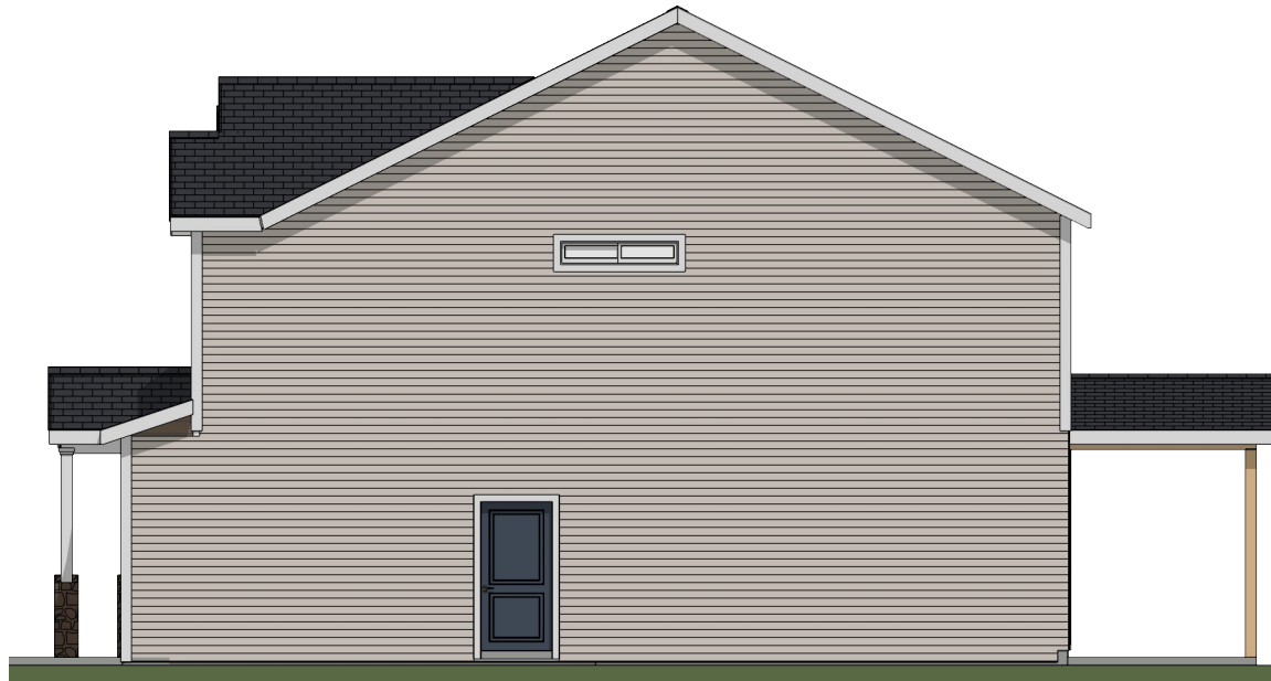
RIGHT ELEVATION
